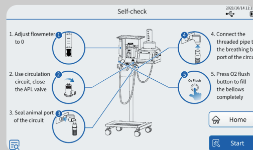
Interfaz de autodiagnóstico
